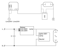
Technische Daten Philips BHL 250 L307 230 240V 50Hz BC2-134
