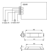
Technische Daten Philips HID-PV m 20 /I CDM HPF 220-240V 50/60Hz für 20W
